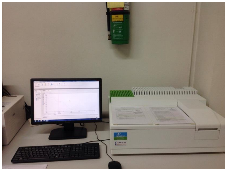
เครื่อง ยูวีวิสิเบิลสเปกโตสโกปี
