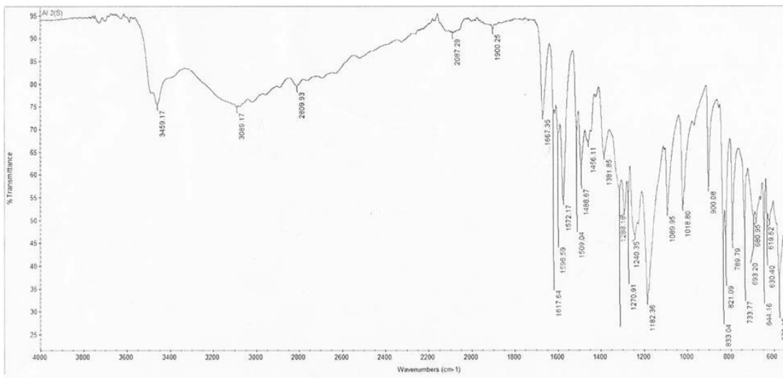
IR spectrum สาร B
