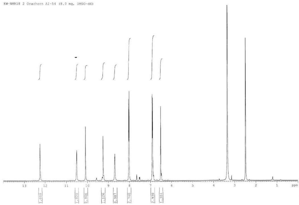
^1\text{H-NMR} spectrum สาร A
