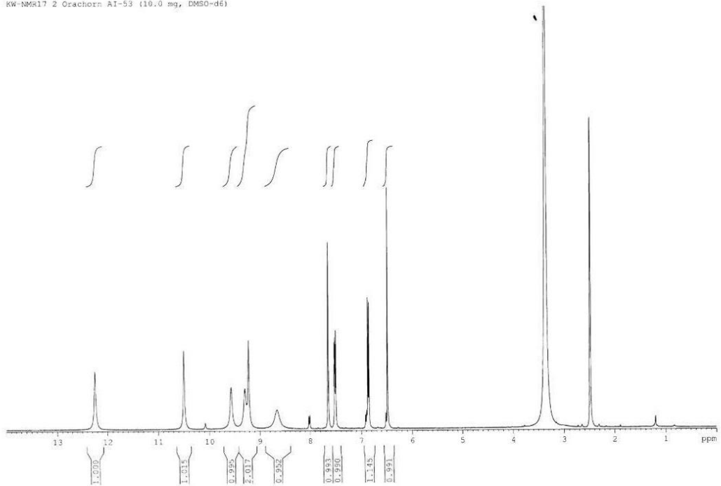
^1\text{H-NMR} spectrum สาร B
