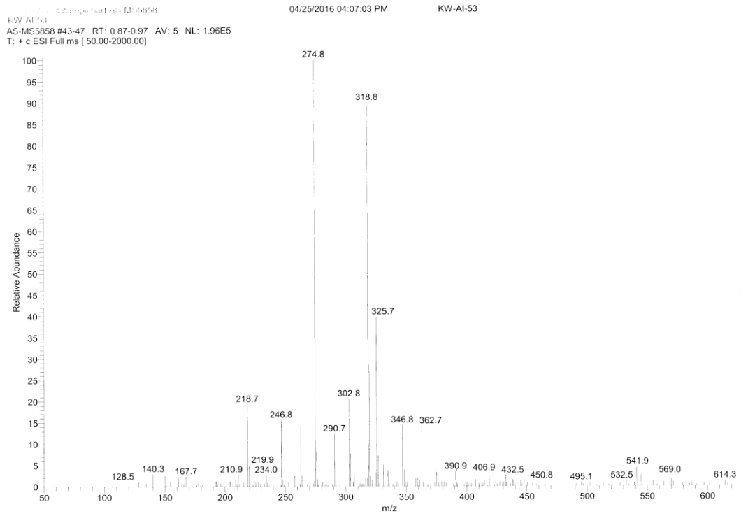
MS spectrum สาร B
