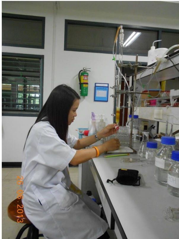
การแยกด้วยคอลัมน์ โครมาโตกราฟี
