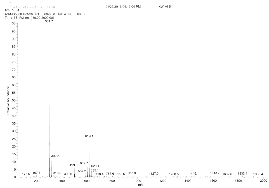
MS spectrum สาร A
