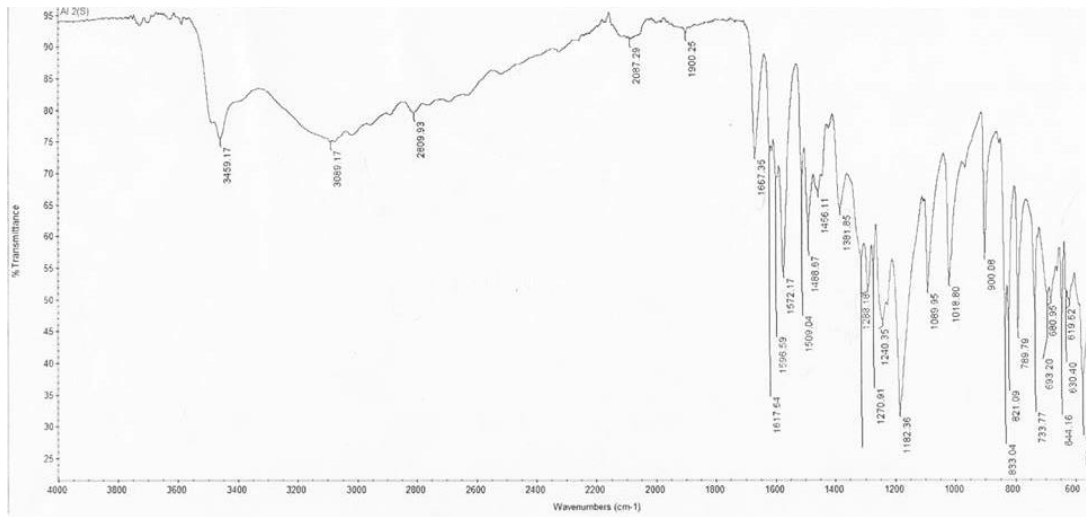
IR spectrum สาร A
