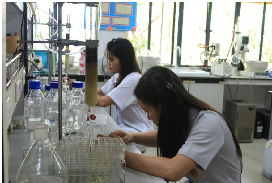
แยกด้วยคอลัมน์โครมาโตกราฟี
